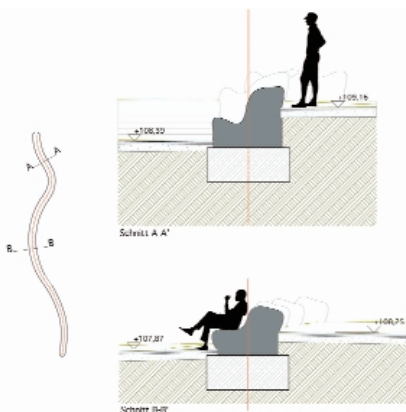
Schnitt durch das vordere und das hintere Ende des Sofas
